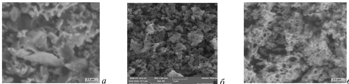
Рис. 1. Микрофотографии образцов \text{La}_2\text{O}_3 - \text{NiO} - \text{MnO} , полученных при различном соотношении «топливо»/( \text{NO}_3^- ) ( a - 0.2 , b - 0.55 (stech), v - 1.2 ). В представленном случае качестве топлива использован глицин
