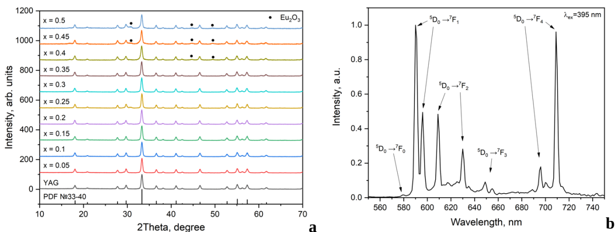
Рисунок 1. Дифрактограммы YAG:xEu (а) и спектр эмиссии образца YAG:0.3Eu (б)
