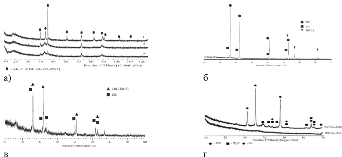
Рисунок 1. Данные РФА синтезированных при 1000\text{--}1300^\circ\text{C} порошков систем: а – \text{Mo} - \text{C} ; б – (\text{Ti-Si-W}) - \text{C} ; в – (\text{Ti-Si-Cr}) - \text{C} ; г – (\text{W-Co}) - \text{C} .
