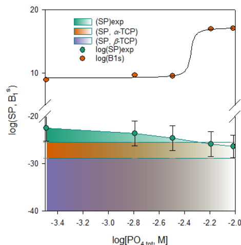
Рисунок. Экспериментальная растворимость (SP) фосфата кальция в растворах K 2 HPO 4 , pH=6–11. 23°C
